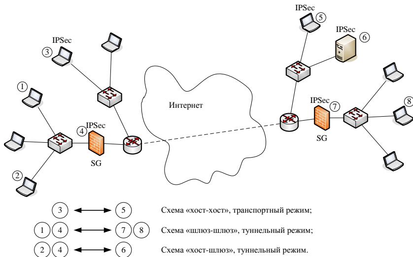
Рисунок 45 – Схемы работы IPSec
