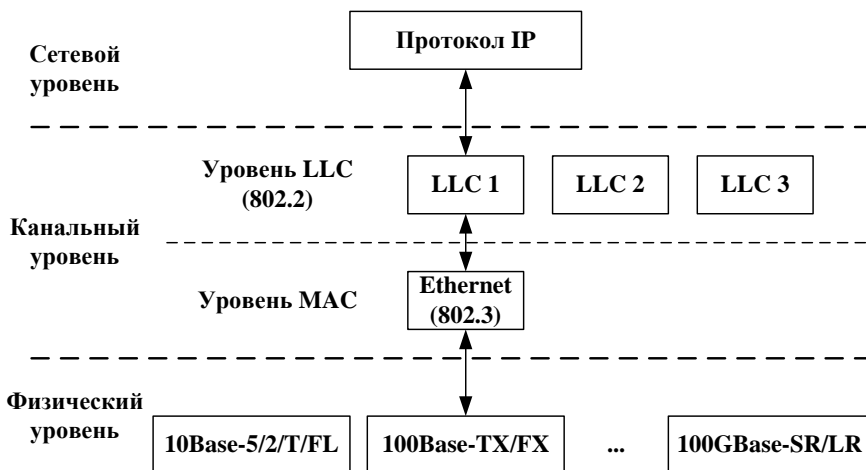
Рисунок 23 – Функциональные уровни технологии Ethernet
