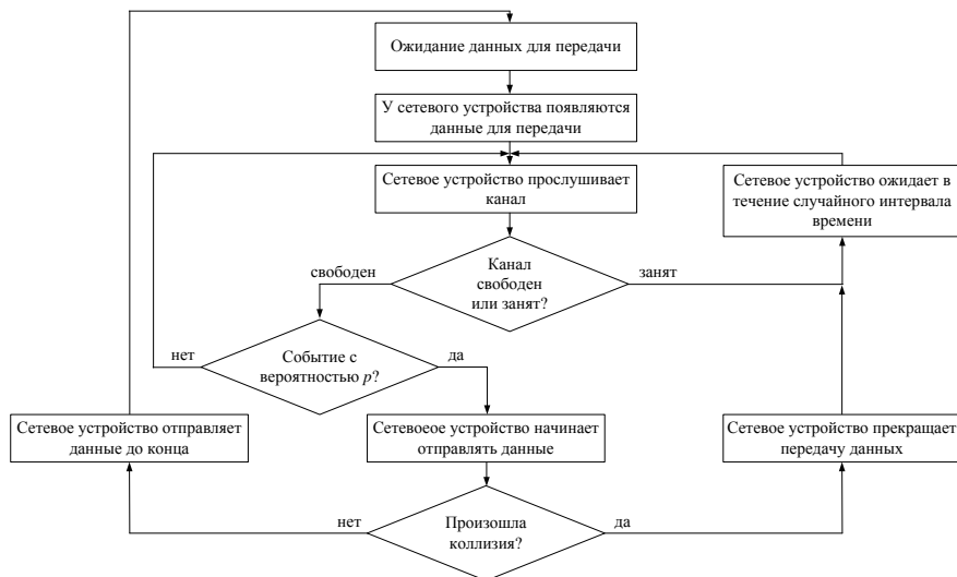
Рисунок 26 – Алгоритм процесса передачи данных сетевым устройством по протоколу CSMA/CD
