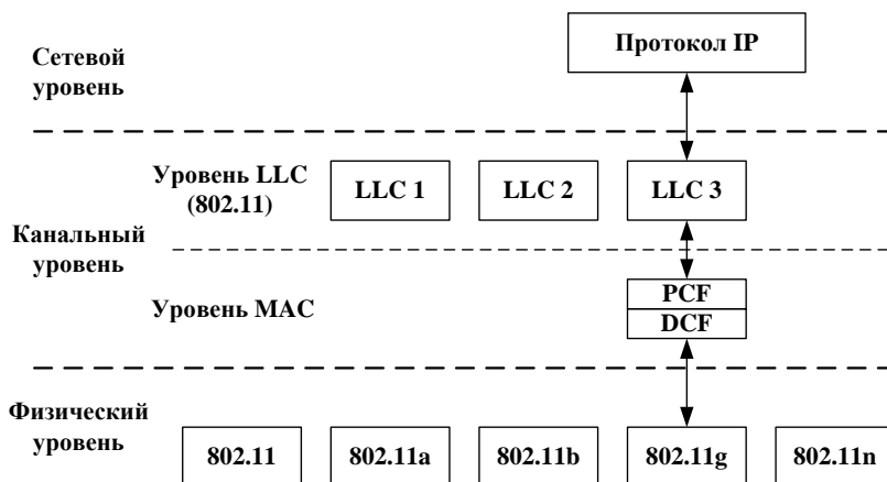
Рисунок 30 – Функциональные уровни технологии 802.11
