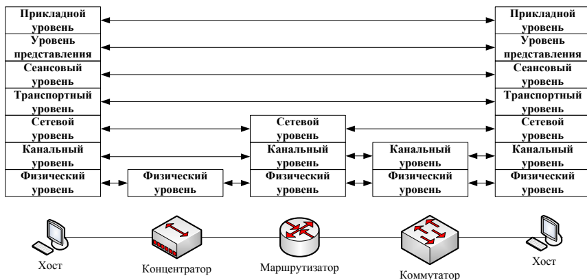
Рисунок 8 – Соответствие функций различных устройств сети уровням модели OSI
