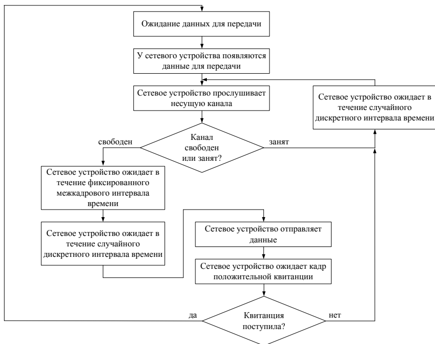
Рисунок 29 – Алгоритм процесса передачи данных сетевым устройством по протоколу CSMA/CA
