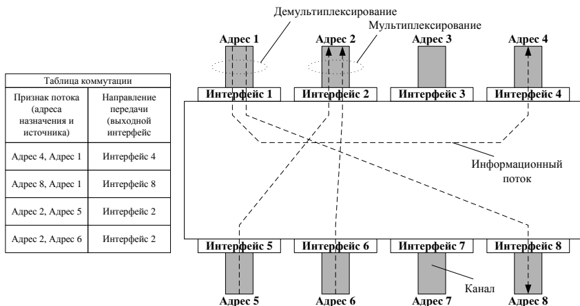
Рисунок 11 – Таблица коммутации
