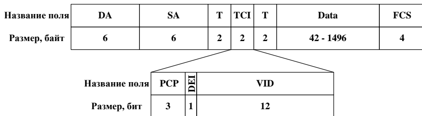
Рисунок 32 – Формат кадра технологии Ethernet с пометкой VLAN
