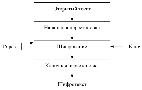
Рисунок 19 – Обобщенная схема шифрования в алгоритме DES
