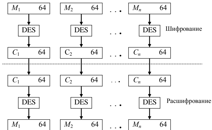
Рисунок 20 – Схема алгоритма DES в режиме электронной кодовой книги
