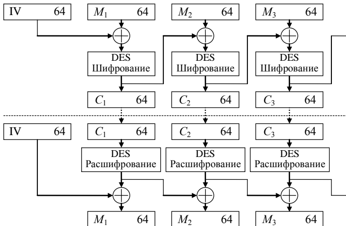
Рисунок 21 – Схема алгоритма DES в режиме сцепления блоков шифра
