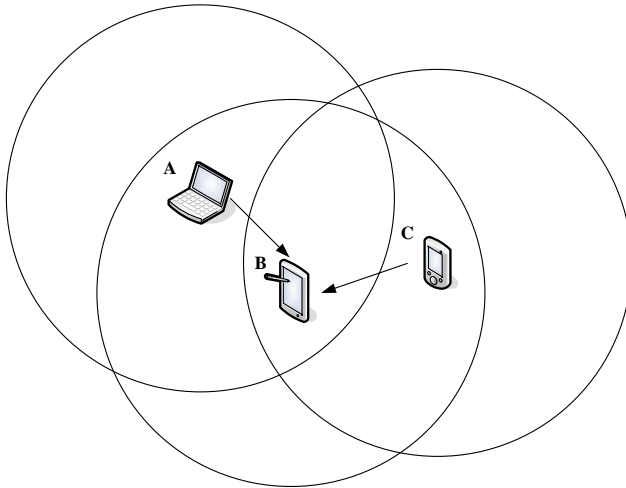
Рисунок 27 – Проблема скрытого сетевого устройства
