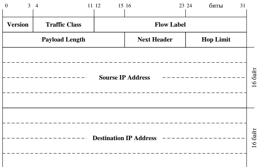
Рисунок 37 – Структура основного заголовка IPv6
