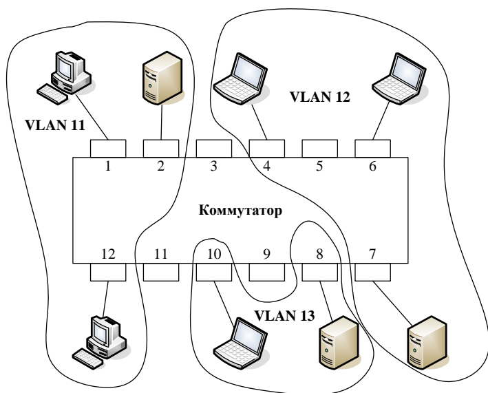
Рисунок 31 – VLAN на основе одного коммутатора
