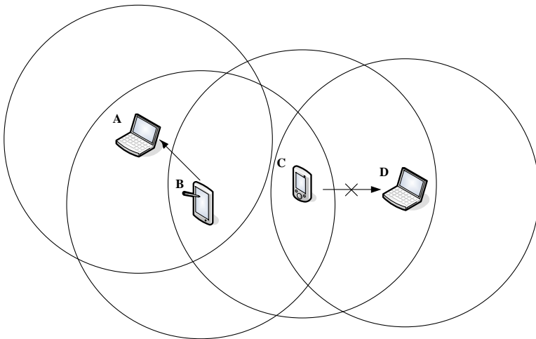
Рисунок 28 – Проблема засвеченного сетевого устройства
