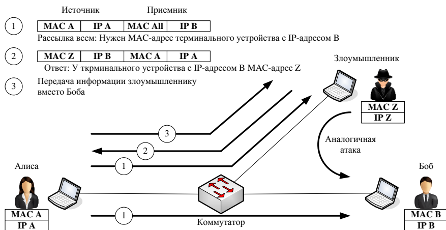
Рисунок 33 – ARP-spoofing
